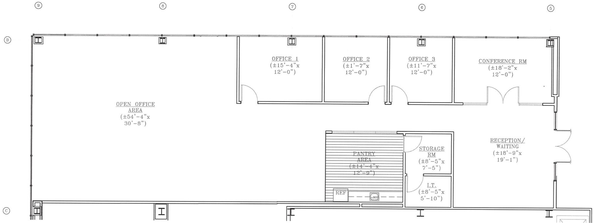
1 FLOOR PLAN SCALE: 1/8" = 1'-0"
